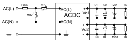
图3:AWH10-10DXXX(双隔离双路)系列典型应用电路
